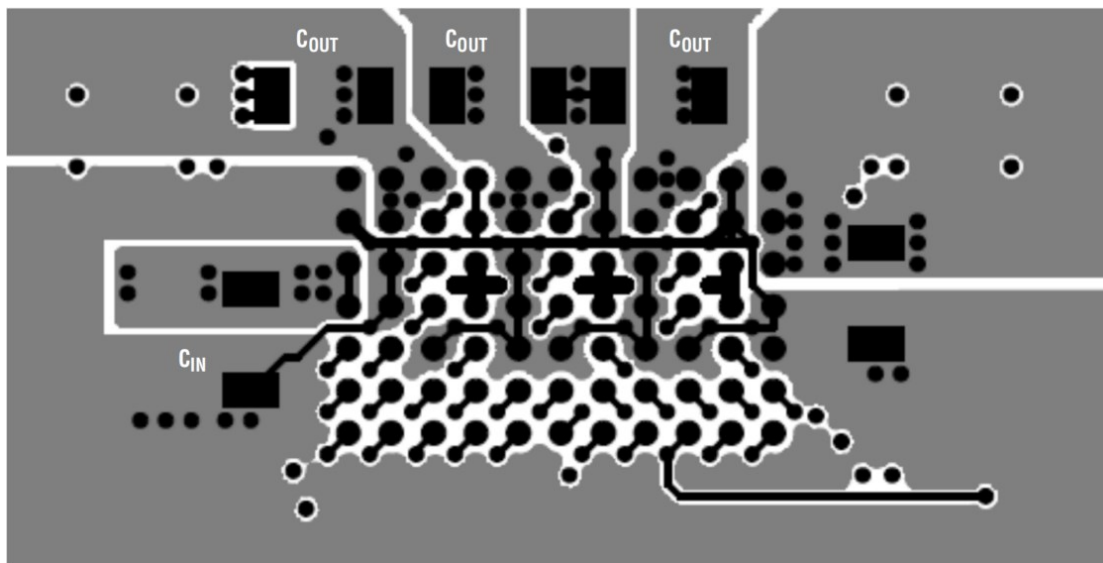
图 7 PCB 布局
